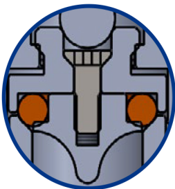
Conjunto de Vedação com Defletor para direcionamento de fluxo
